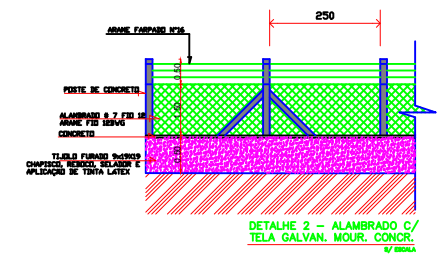
Detalhe 1,2- Alamedro c/ tela Galvanizada Mourão Concreto
