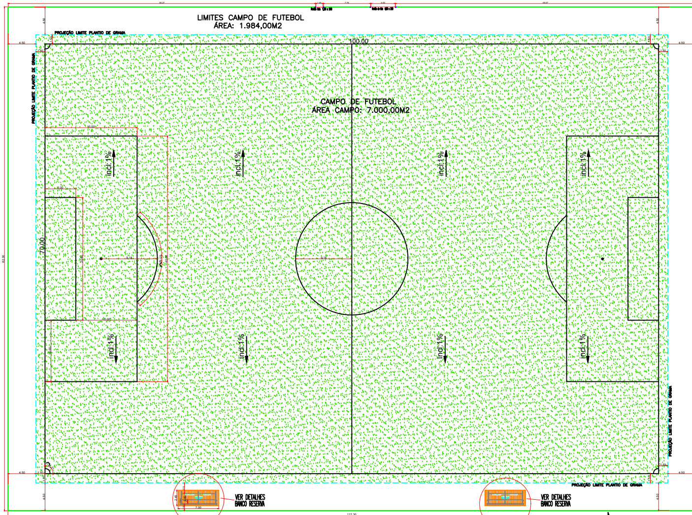
PLANTA BAIXA - IMPLANTAÇÃO ESCALA: 1/50
